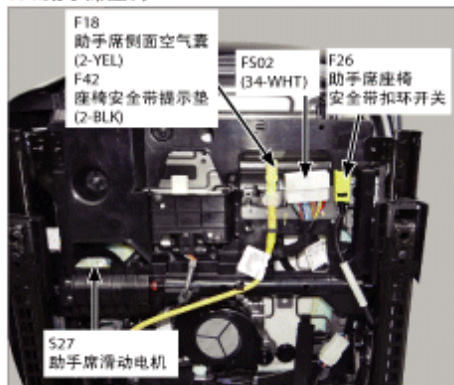
131.助手席座椅
