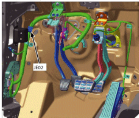
127.防火板左侧
